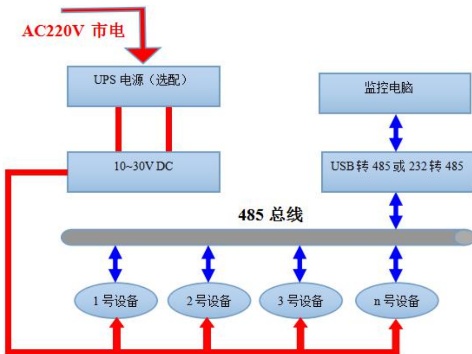
系统方案图
